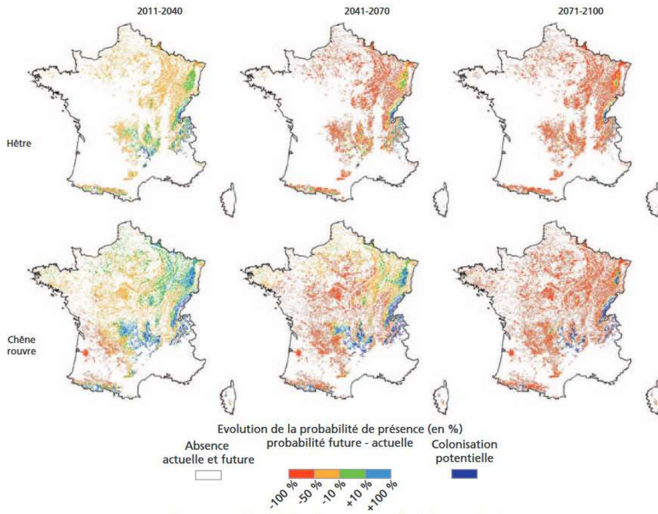
Evolution prévisible de la distribution potentielle du hêtre et du chêne rouvre à partir du modèle +4,2°C (Modèle HadCM3 scénario -A2) (source : IF – Forêt et changements climatiques : apports des données d’inventaire IGN - 2014)
